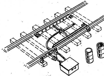
48-137 Flange Lubricator
